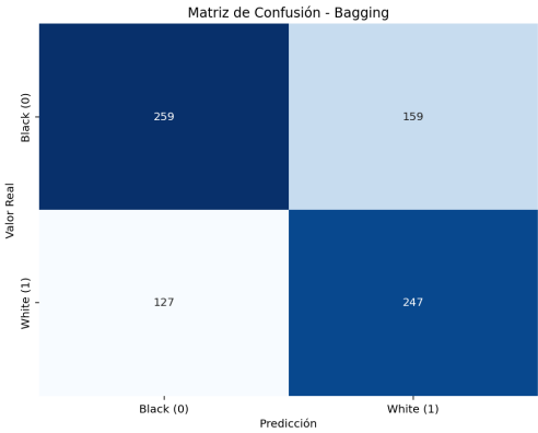
Figura 19: Matriz de confusión para bagging
